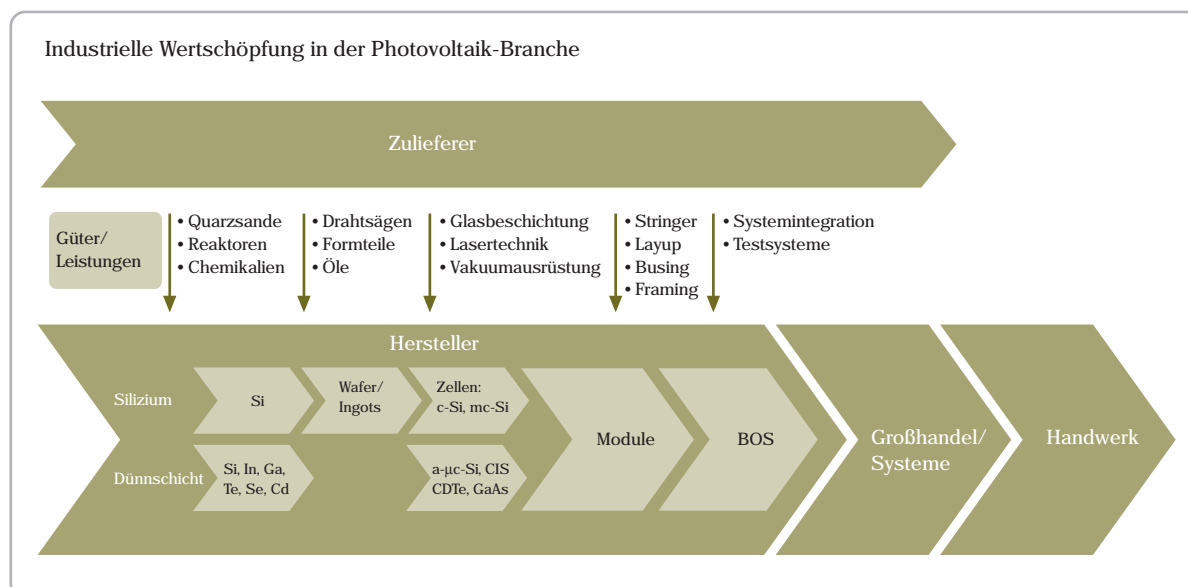
Überblick über die industrielle Wertschöpfung in der Photovoltaikbranche
