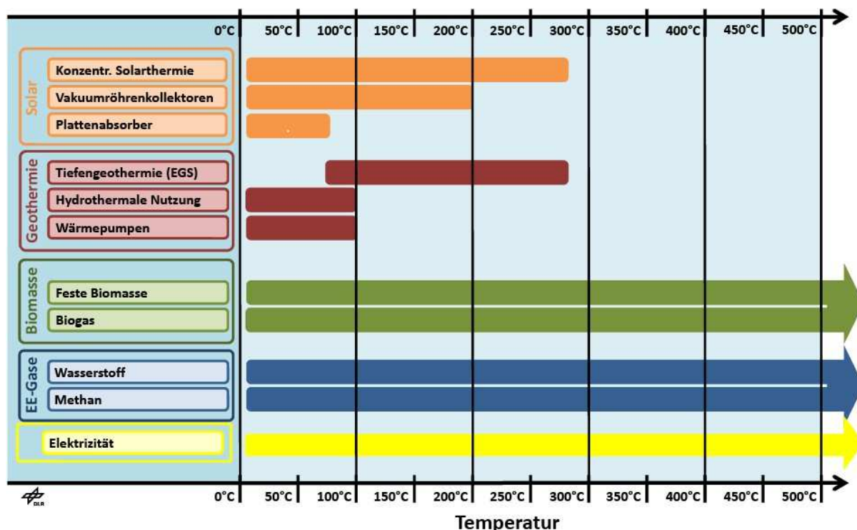
Abbildung 6: Erzielbare Temperaturen der unterschiedlichen Erneuerbaren Energieträger (Quelle: DLR 2016: Prozesswärme für die Industrie: Einsatz erneuerbarer Technologien abhängig von Temperaturanforderungen).
