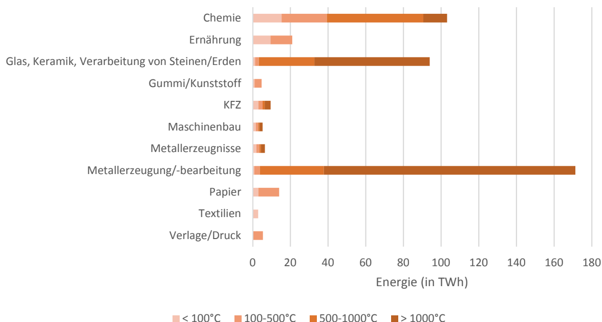
Abbildung 2: Temperaturniveaus der Prozesswärme in relevanten Branchen (Quelle: ifeu / DLR 2010: Prozesswärme im Marktanzreizprogramm).
