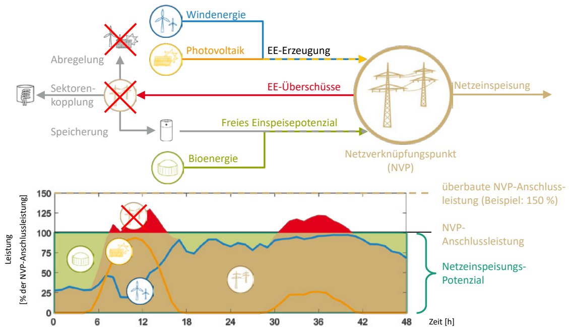
Abb. 1: Schematische Darstellung der gemeinschaftlichen NVP-Nutzung und Überbauung
