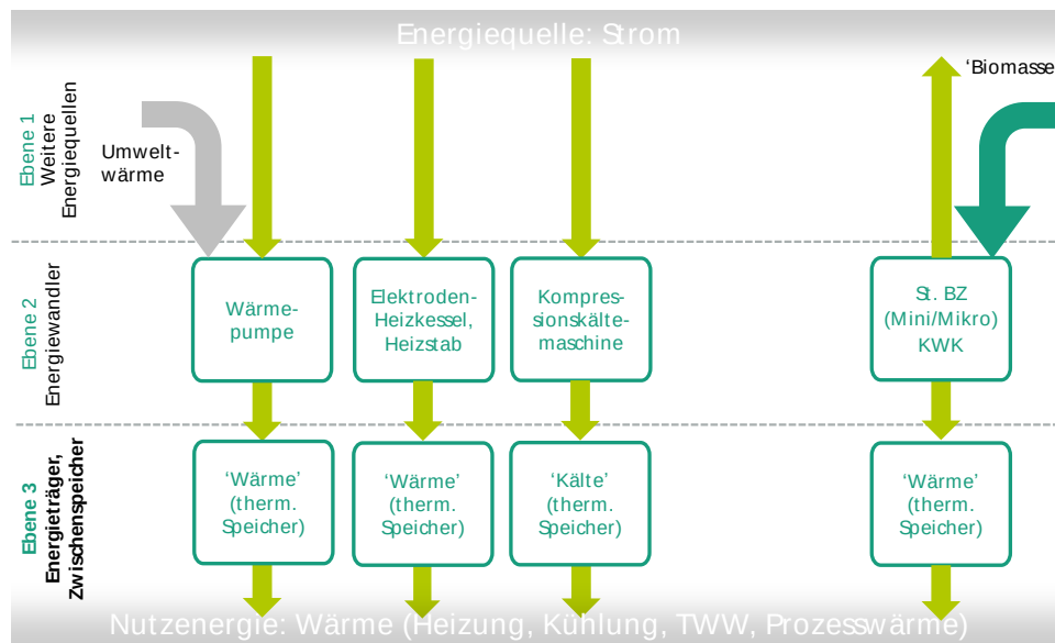
Abbildung 10: 3.3 Interaktionsanalyse Strom/Wärme
