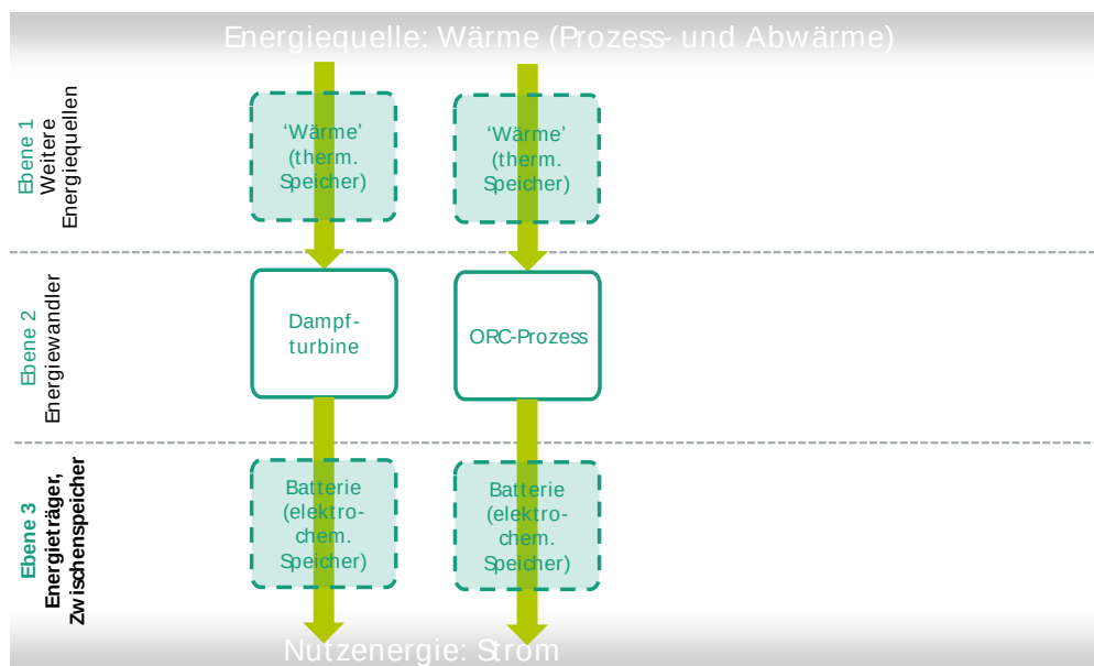
Abbildung 11: Interaktionsanalyse Wärme/Strom
