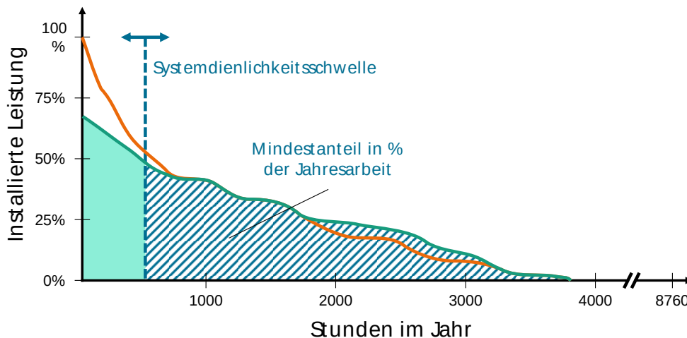
Abbildung 23: Definition der Systemdienlichkeitsschwelle und systemdienliche Mindestanteil (Jansen 2017)
